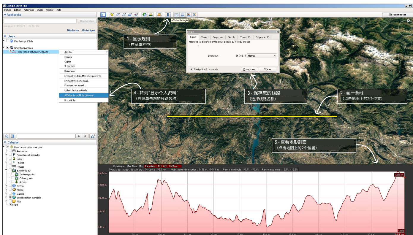
比利牛斯山脉的地形剖面图 © Google Earth。
