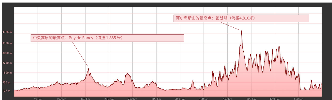
中央高原和阿尔卑斯山之间 650 公里的地形剖面 © Google Earth。
