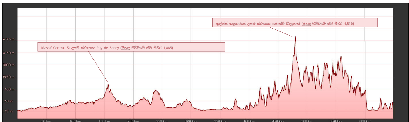
Massif Central සහ Alps © Google Earth අතර කිලෝමීටර් 650ක භූලක්ෂණ පැතිකඩ.
