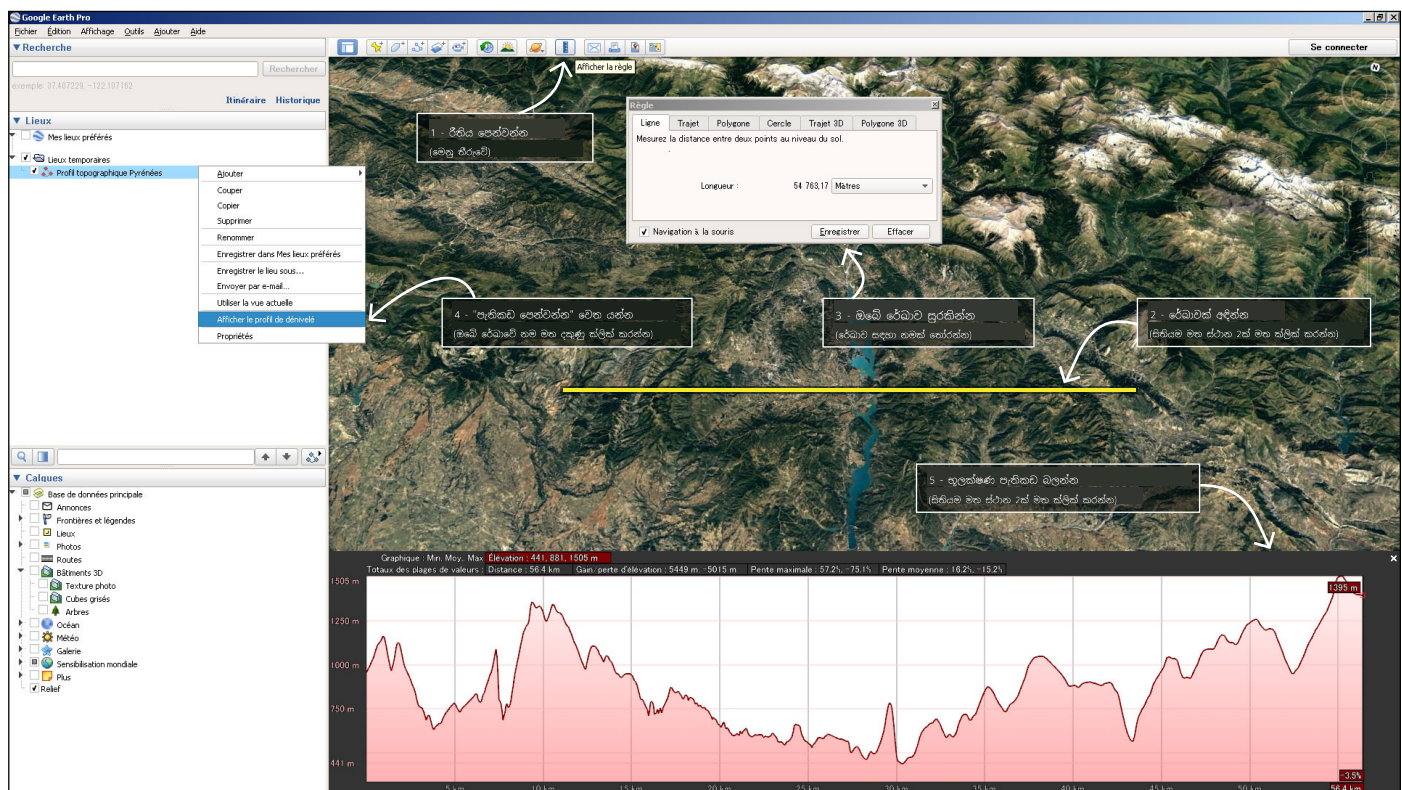
Pyrenees © Google Earth හි භූලක්ෂණ පැතිකඩ.
