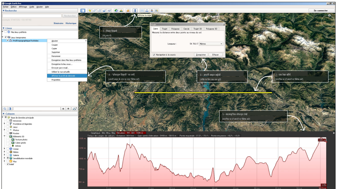
पाइरेनीज़ की स्थलाकृतिक प्रोफ़ाइल © Google Earth।
