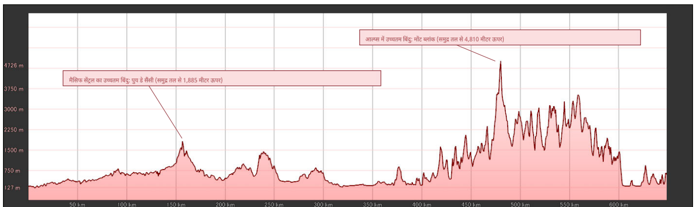
मैसिफ़ सेंट्रल और आल्प्स के बीच 650 किलोमीटर की स्थलाकृतिक प्रोफ़ाइल © Google Earth।
