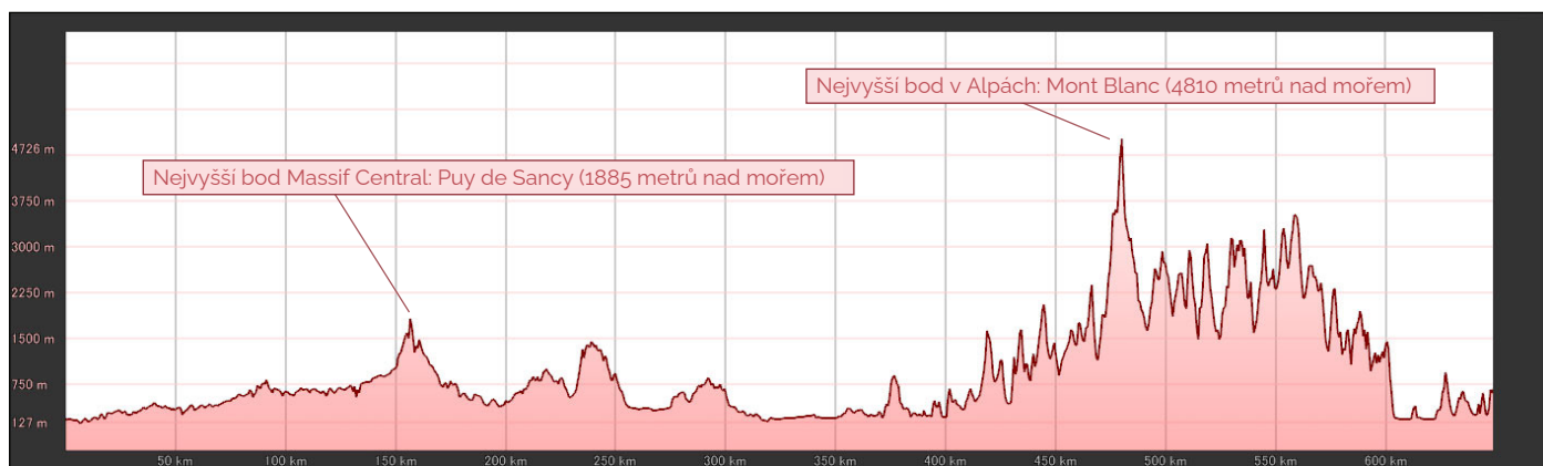
Topografický profil 650 kilometrů mezi Massif Central a Alpami © Google Earth.
