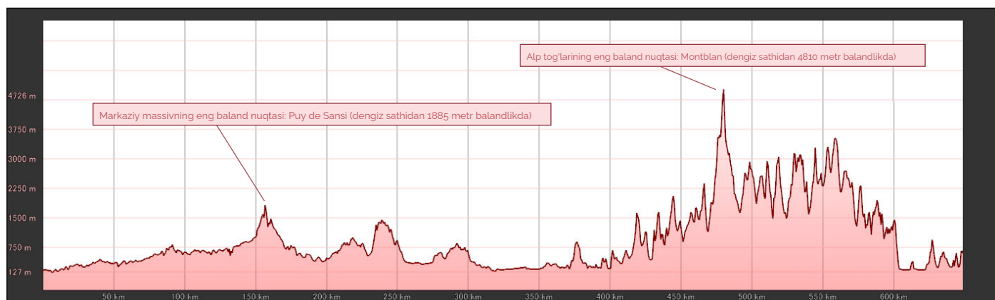
Markaziy massiv va Alp tog'lari orasidagi 650 kilometrlik topografik profil © Google Earth.
