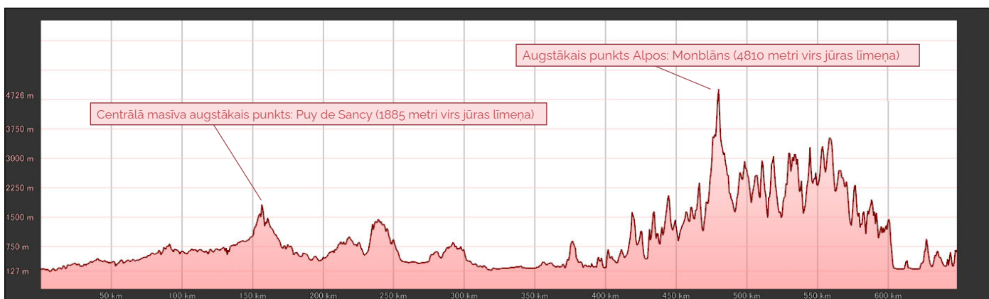
Topogrāfiskais profils 650 kilometru garumā starp Centrālo masīvu un Alpiem © Google Earth.
