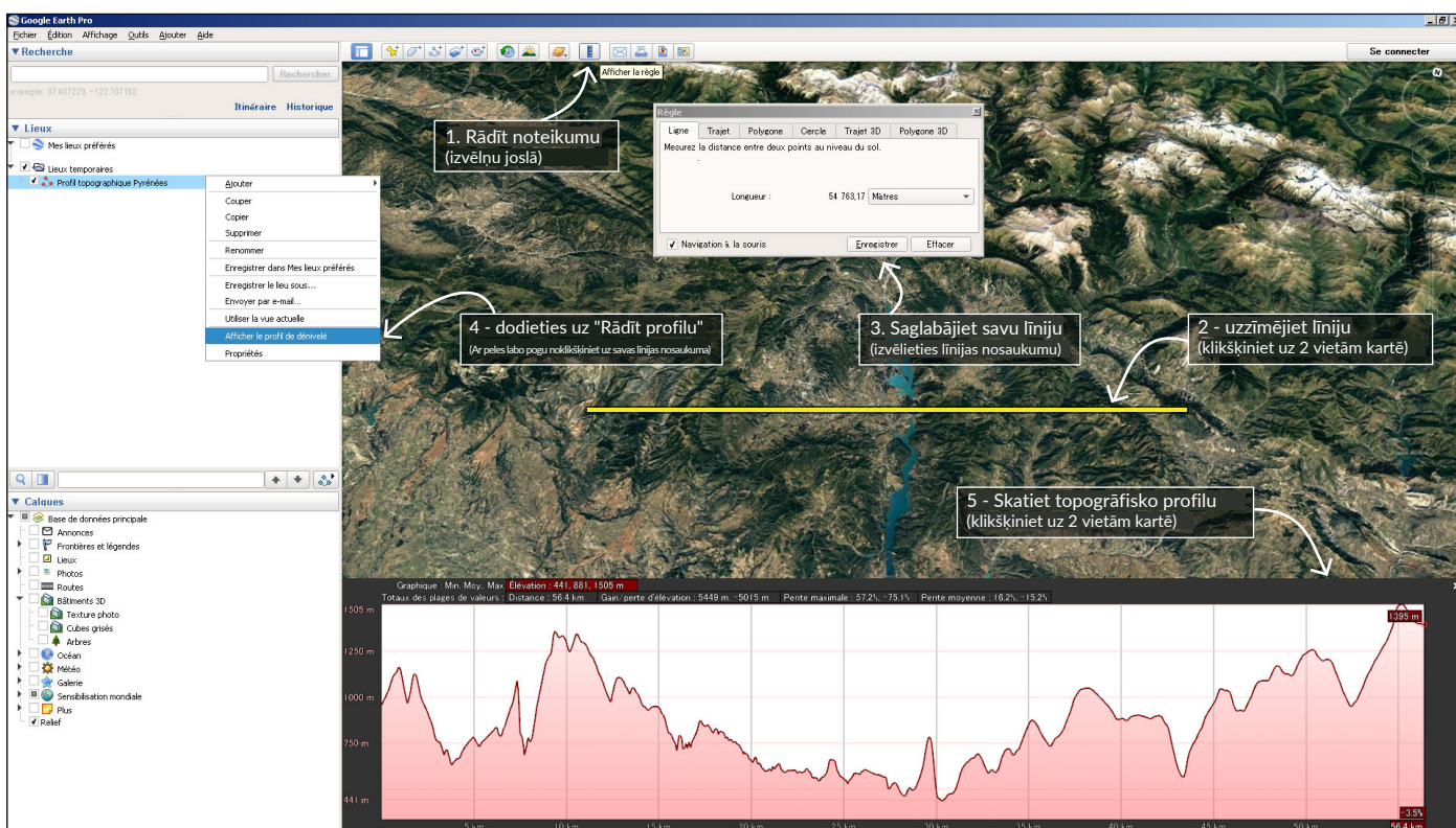
Pyreneju topogrāfiskais profils © Google Earth.
