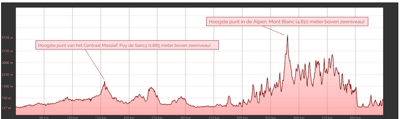
Topografisch profiel van 650 kilometer tussen het Centraal Massief en de Alpen © Google Earth.
