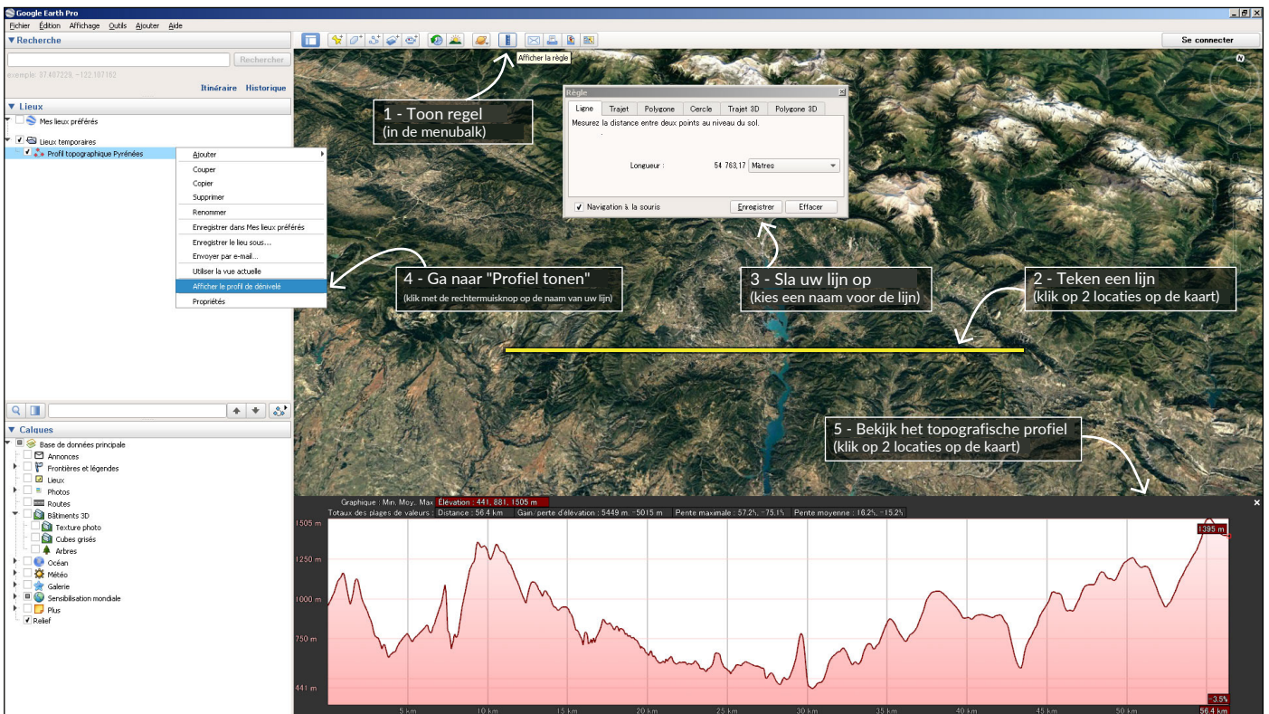
Topografisch profiel van de Pyreneeën © Google Earth.
